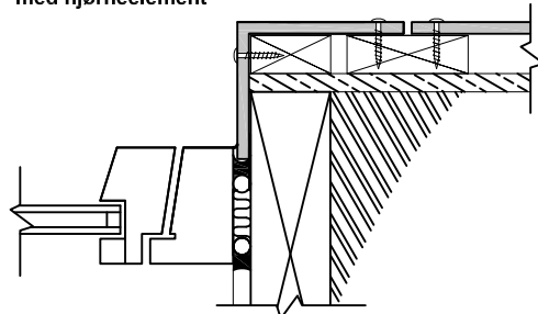
Horizontalsnitt Eksempel på vindusløsning med hjørneelement
