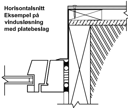
Horizontalsnitt Eksempel på vindusløsning med platebeslag
